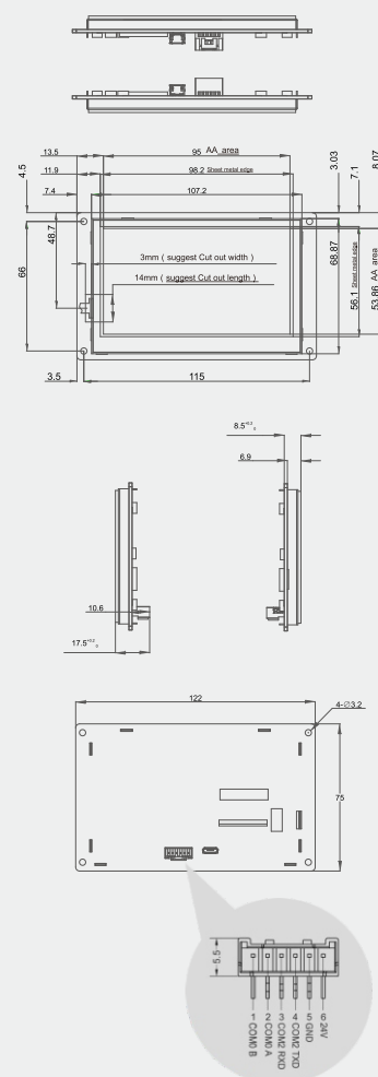
尺寸图 (单位:mm)
